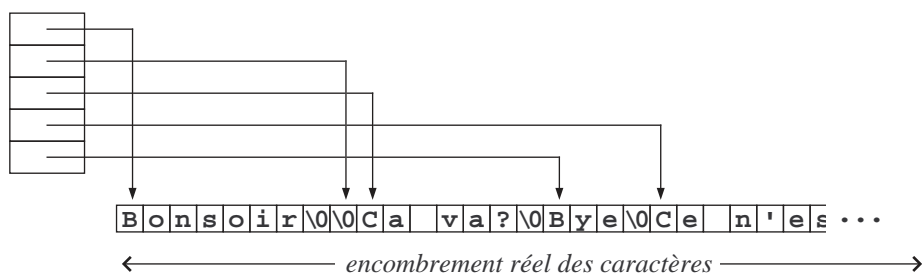
FIGURE 14 – Tableau de chaînes de caractères
