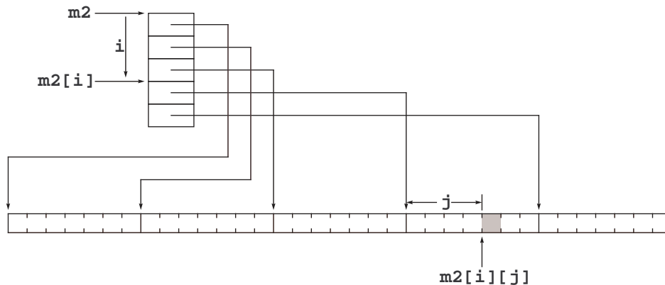
FIGURE 11 – Tableau bidimensionnel réalisé avec un tableau de pointeurs
